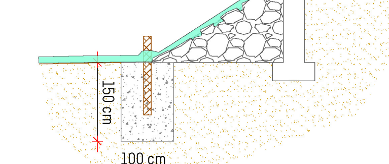
sezione nord-sud
