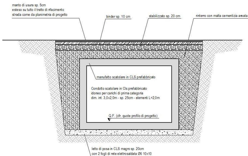
FIGURA 8-4 – INTERVENTO DI PROGETTO, SEZIONE TIPOLOGICA 5 “CANALE IN CONDOTTO PREFABBRICATO IN CALCESTRUZZO ARMATO A SEZIONE RETTANGOLARE”
