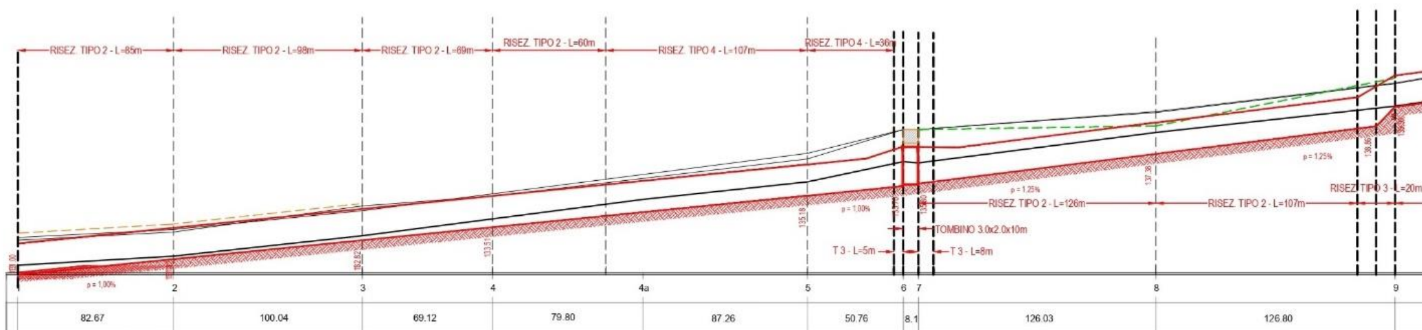
FIGURA 7-3 – RIO ENZOLA, PROFILO LONGITUDINALE DI PROGETTO, TRATTO DA SEZ. 9 A SEZ. 0
