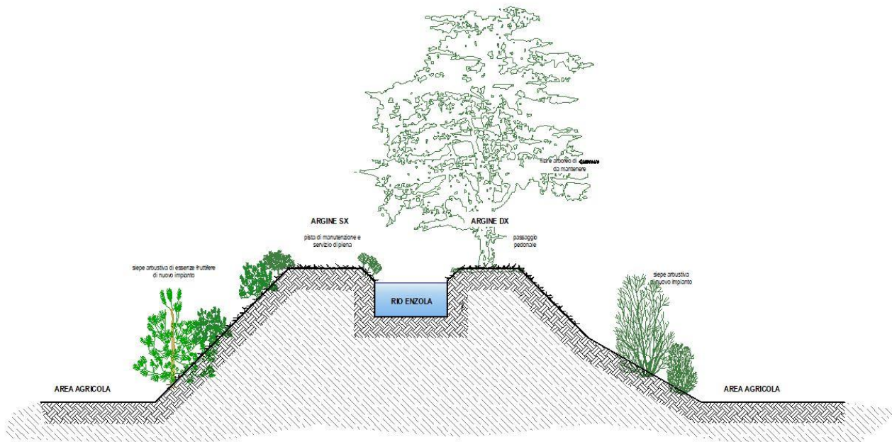
FIGURA 8-7 – RIO ENZOLA: SISTEMAZIONE AMBIENTALE TIPO NEI TRATTI DI SALVAGUARDIA DELLA VEGETAZIONE ARBOREA
