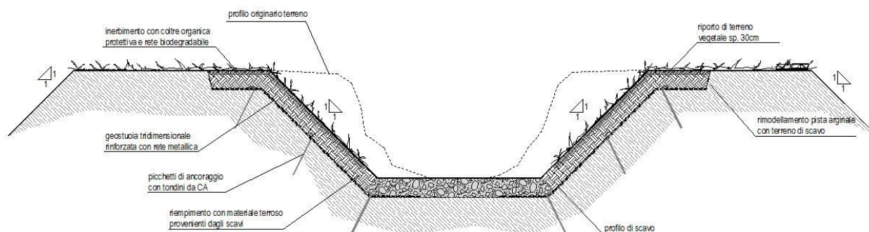
FIGURA 8-1 – INTERVENTO DI PROGETTO, SEZIONE TIPOLOGICA 2 "CANALE INERBITO"
