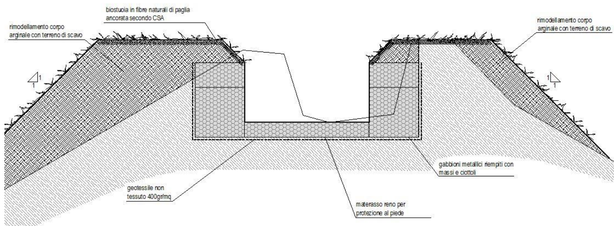
FIGURA 8-3 – INTERVENTO DI PROGETTO, SEZIONE TIPOLOGICA 4 “CANALE IN GABBIONI”
