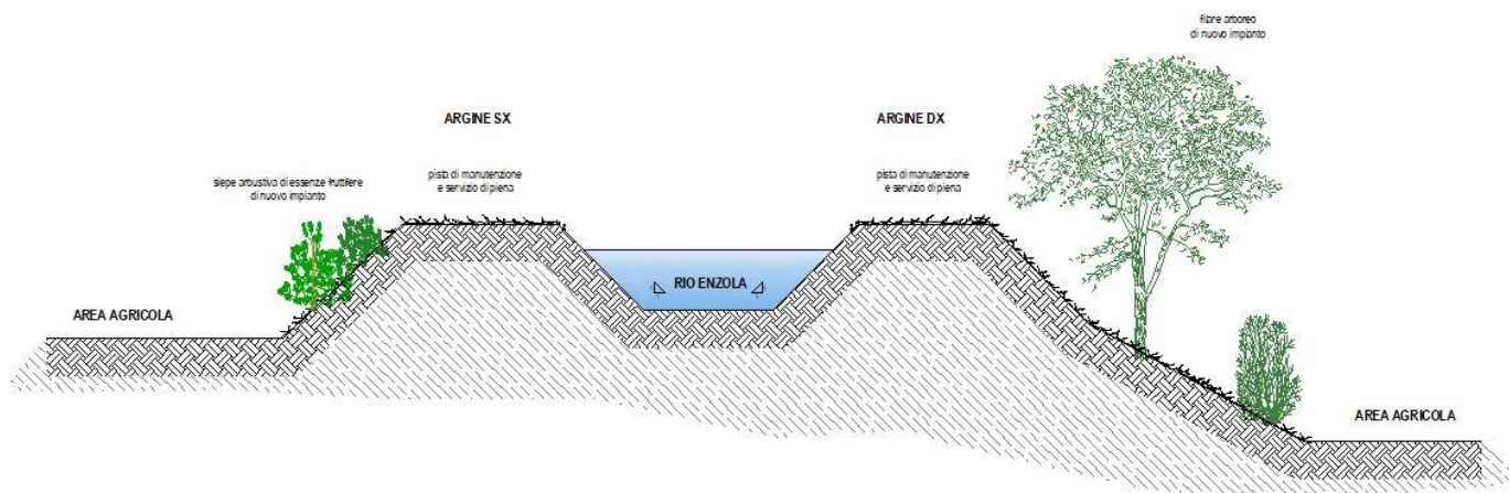
FIGURA 8-6 – RIO ENZOLA: SISTEMAZIONE AMBIENTALE TIPO NEI TRATTI DI NUOVA REALIZZAZIONE
