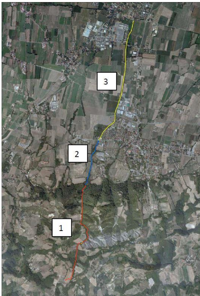
FIGURA 5-2 – ANALISI MORFOLOGICA RIO ENZOLA, SUDDIVISIONE IN TRATTI OMOGENEI (PROGETTO LIFE RII)
