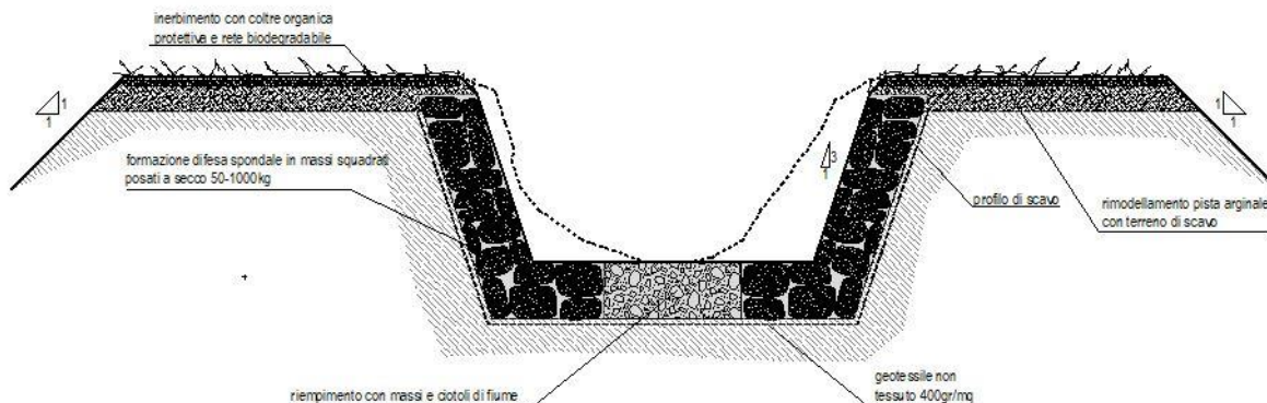
FIGURA 8-2 – INTERVENTO DI PROGETTO, SEZIONE TIPOLOGICA 3 “CANALE IN PIETRAMME SPACCATO A SECCO”
