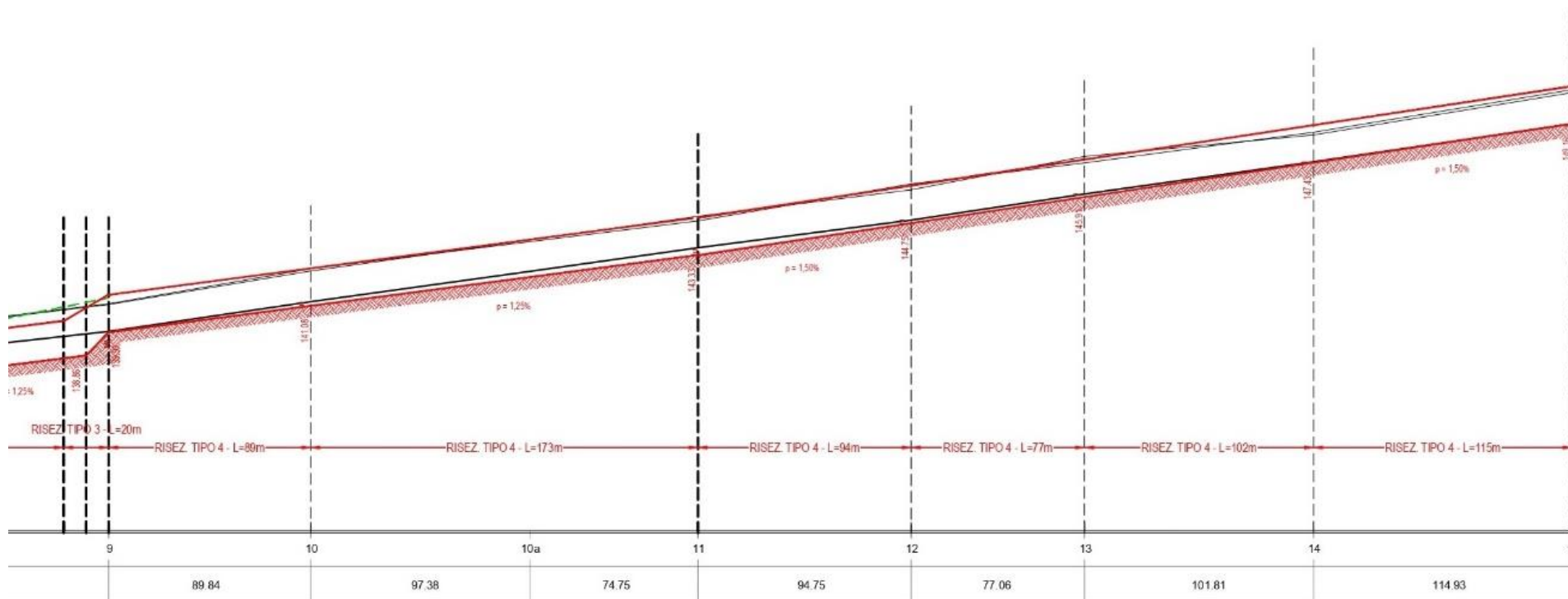
FIGURA 7-2 – RIO ENZOLA, PROFILO LONGITUDINALE DI PROGETTO, TRATTO DA SEZ. 15 A SEZ. 8.8
