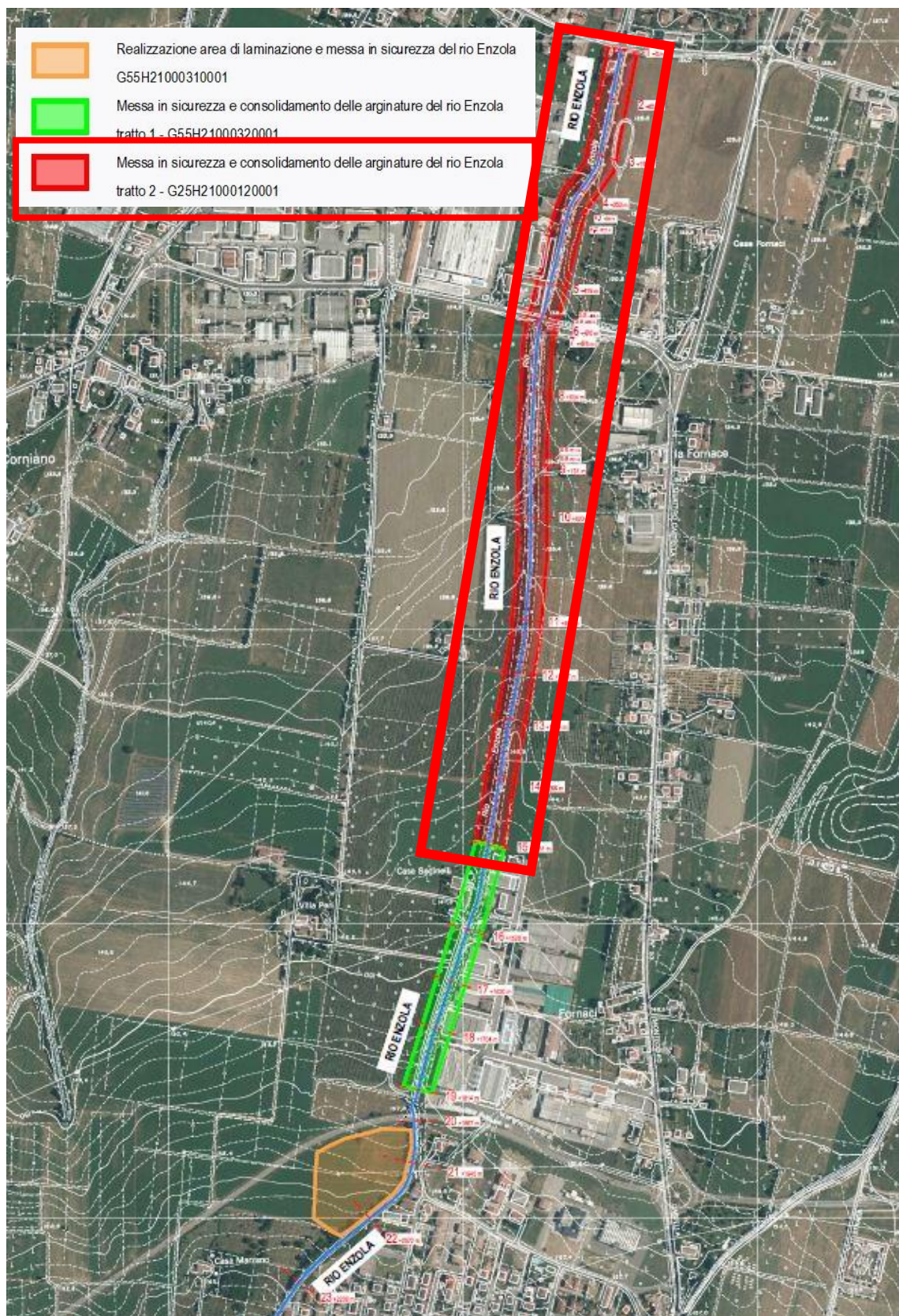
FIGURA 4-1 – ANALISI MORFOLOGICA RIO ENZOLA, INDIVIDUAZIONE AREA DI INTERVENTO
