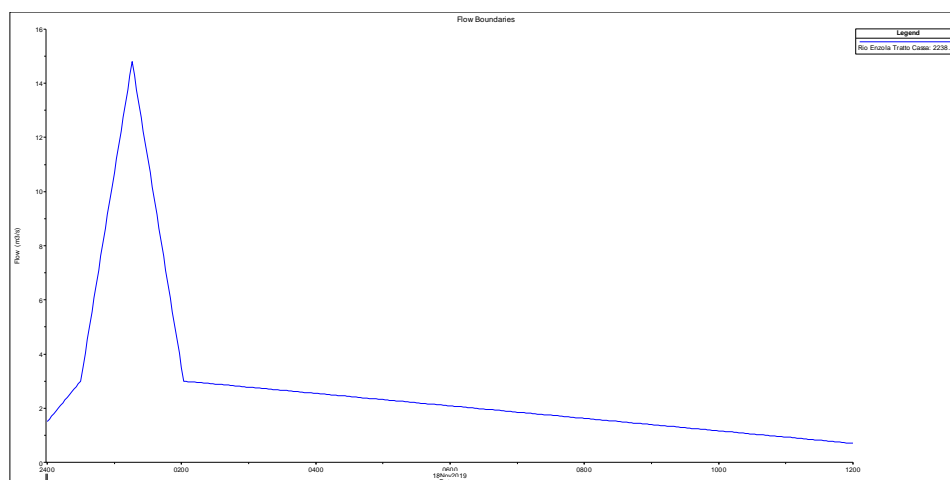
FIGURA 6-1 – RIO ENZOLA, IDROGRAMMA SIMULATO PER UN TEMPO DI RITORNO PARI A 200 ANNI
